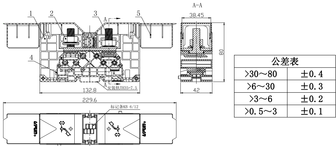
外型尺寸
